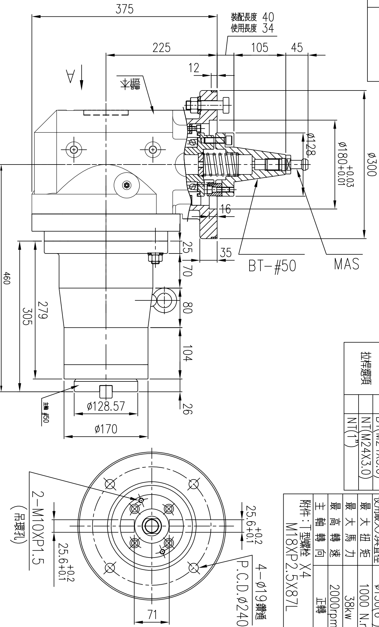
HE73外型圖
